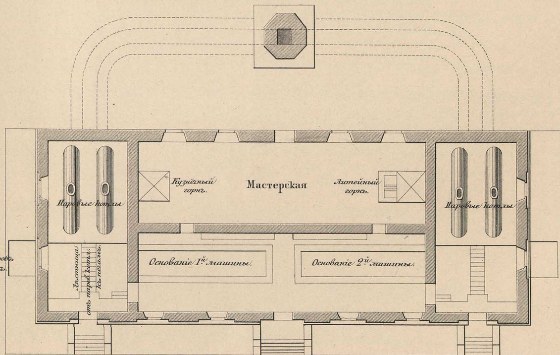
Масштабъ къ фасаду и плану.
